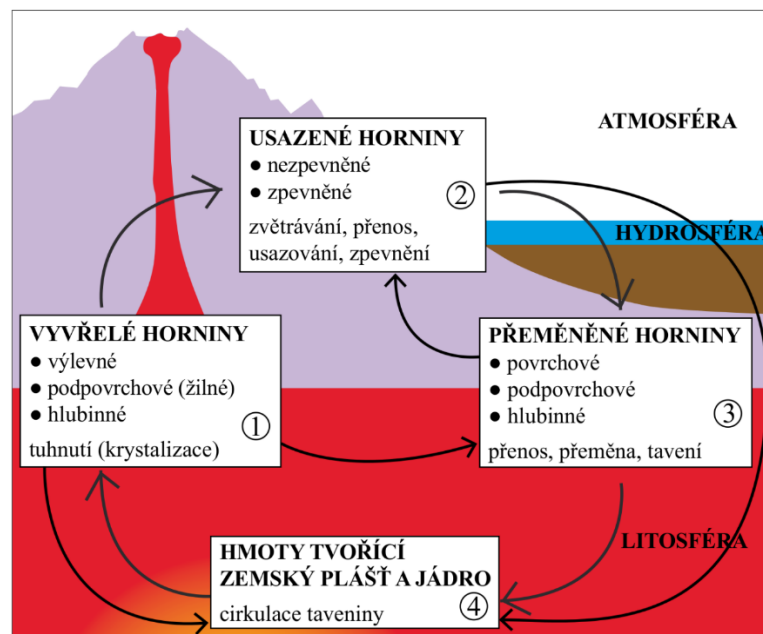
schéma – horninový cyklus
